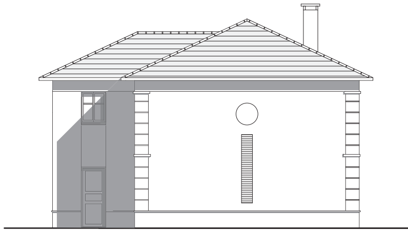
FAÇADE ARRIÈRE - OUEST
