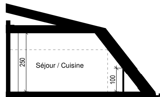
COUPE A-A
