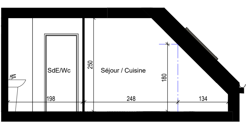
COUPE A-A
