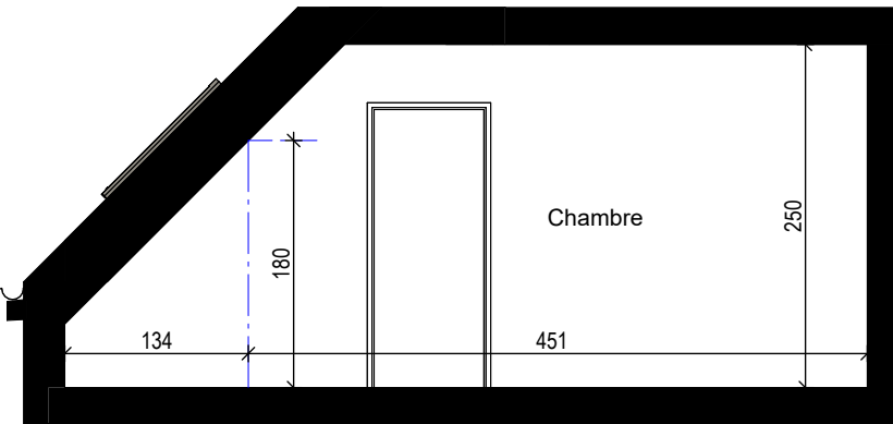
COUPE A-A
