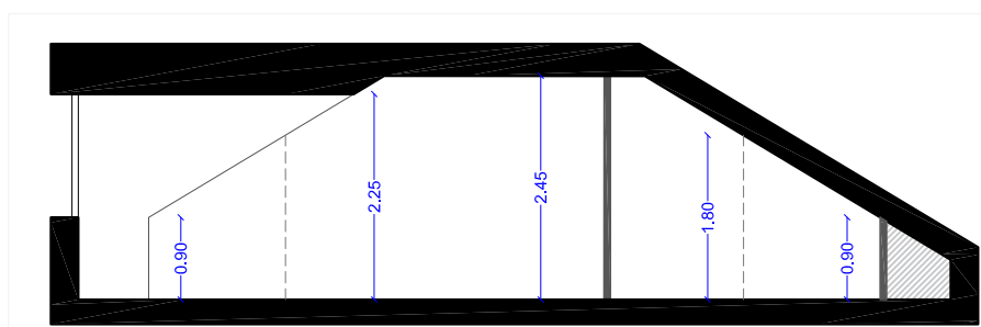
Coupe de principe du logement
